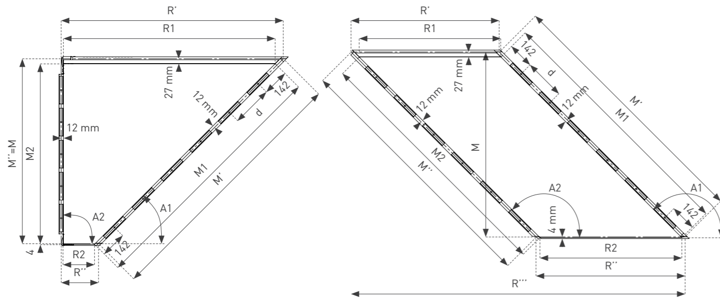
R'' min = 200 mm, R' max = 6400 mm, A1 = 45° to 89.9°, A2 = 90°
